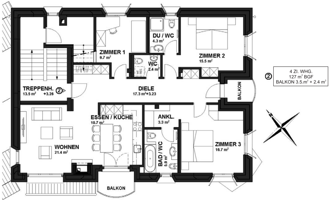
Chesa Lodola Obergeschoss 1:100
